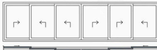
Coulissant à levage 6 vantaux, 3 rails
