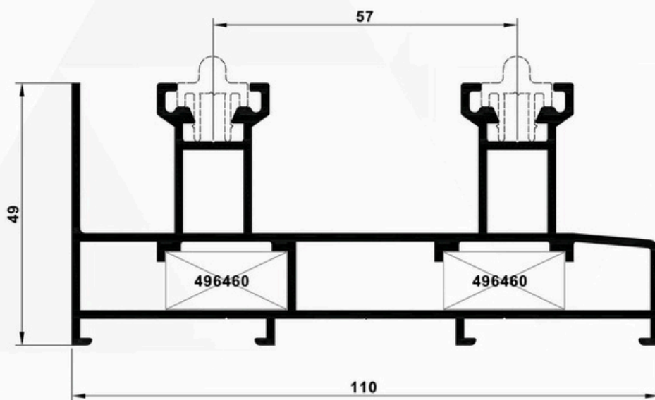
Réf. 8964/640 Dormant 110 mm 2 rails
