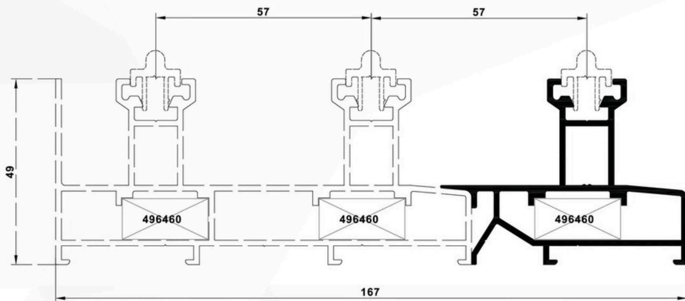
Réf. 21015/640 Complément Dormant 03 Rails
