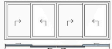
Coulissant à levage 4 vantaux, 2 rails
