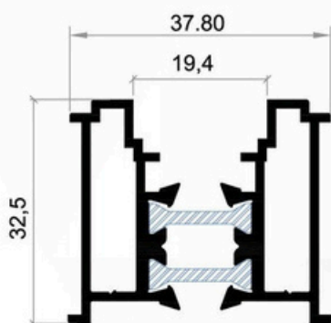
Réf. 8962M/640 Profil de Jonction
