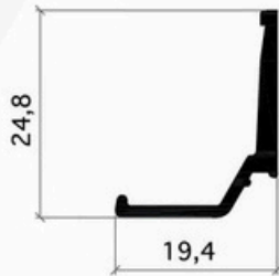
Réf. 8485/640 Parclose
