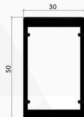
Réf. PL600.42 Renfort
