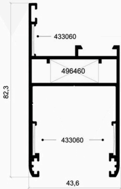
Réf. 8951/640 Ouvrant périmétral
