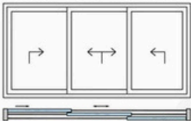
Coulissant à levage 3 vantaux, 3 rails
