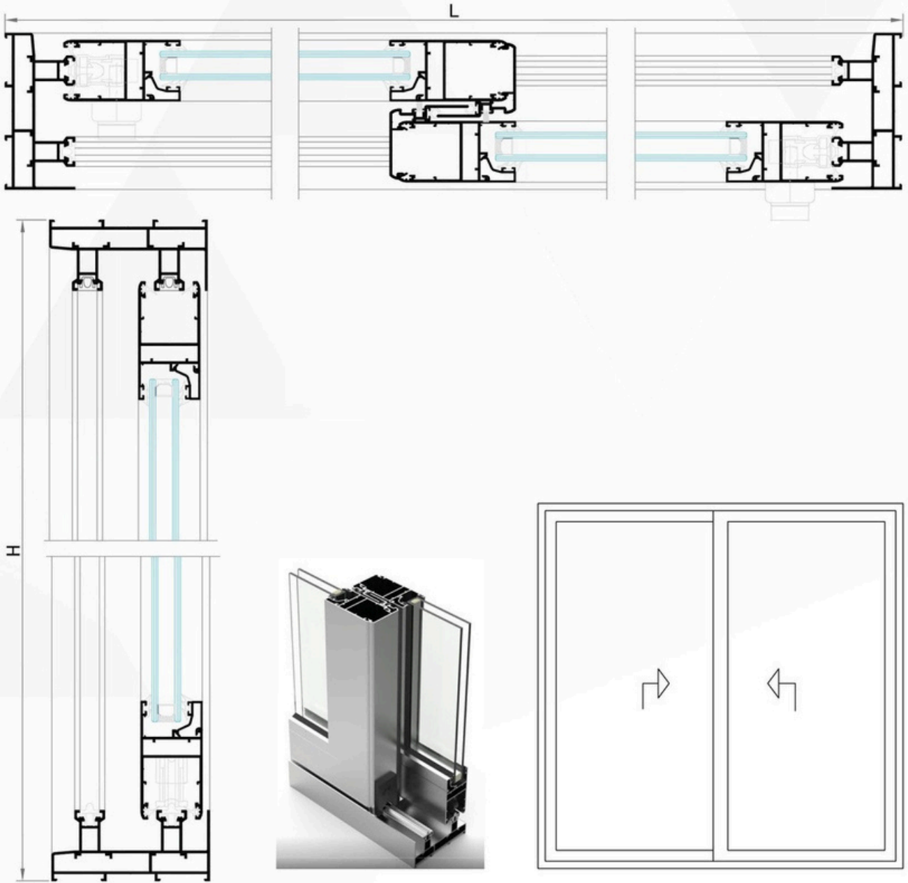
Coulissant 2 vantaux, 2 rails
