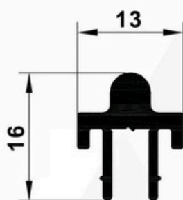
Réf. 895401/ANN/640 Rail anodisé naturel
