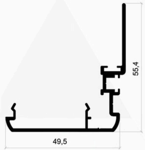
Réf. 8952/640 Chicane
