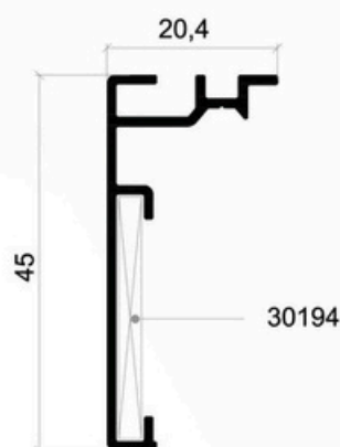
Réf. 2877/650 Couvre joint droit 45mm
