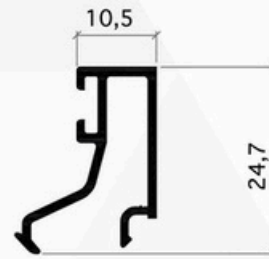
Réf. 8207/640 Parclose
