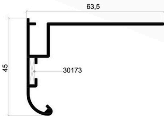
Réf. 2850/650 Couvre joint arrondi 45 mm
