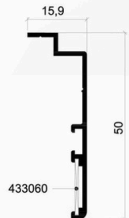
Réf. 8630/640 Couvre joint 50mm
